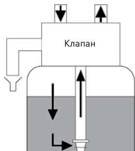
РАБОЧИЙ РЕЖИМ C0
