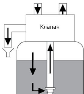
НАГНЕТАНИЕ ДАВЛЕНИЯ C4
