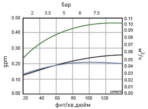
Инжектор «H» (светло-фиолетовый) Для баков диаметром 9 дюймов
