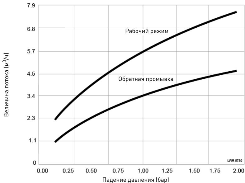
ЗАВИСИМОСТЬ ВЕЛИЧИНЫ ПОТОКА ОТ ПАДЕНИЯ ДАВЛЕНИЯ
