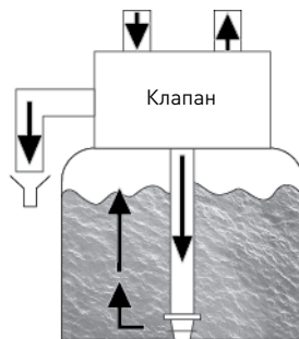
ОБРАТНАЯ ПРОМЫВКА C1
