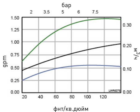
Инжектор «K» (розовый) Для баков диаметром 12 дюймов
