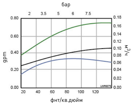
Инжектор «H» (светло-фиолетовый) Для баков диаметром 9 дюймов
