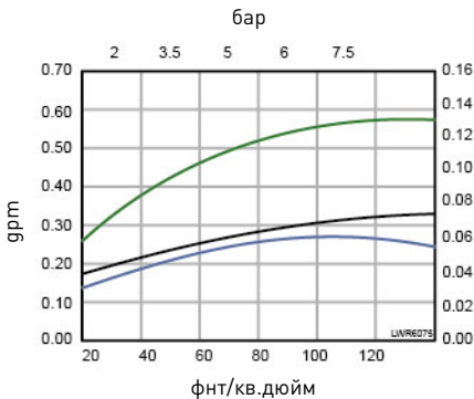
Инжектор «G» (каштановый) Для баков диаметром 8 дюймов
