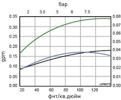
Инжектор «G» (каштановый) Для баков диаметром 8 дюймов
