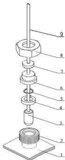
Рис.3. Схема сборки узла УФ датчика.
